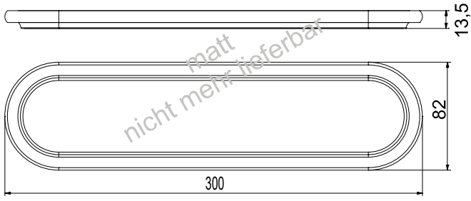
Riva klar/clair BA38xx816 mattiert/opaue BA38xx817
