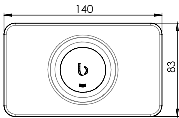
Chic 22 Klar/clair BA21xx805 Mattiert/opaque BA21xx806 Tritan BA21xx807
